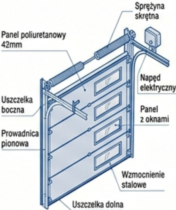
Przekrój konstrukcyjny bramy segmentowej
